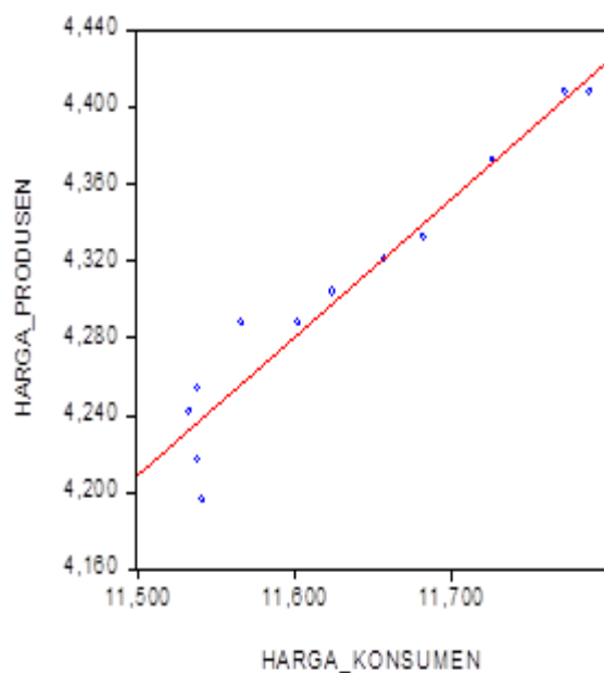
Gambar 1. Diagram Pencar Uji Heterokedastisitas
